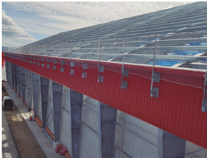
Nave Puerto Exterior de Metalúrgicas del Deza, S.A. (Metaldeza) Arteixo (A Coruña)
